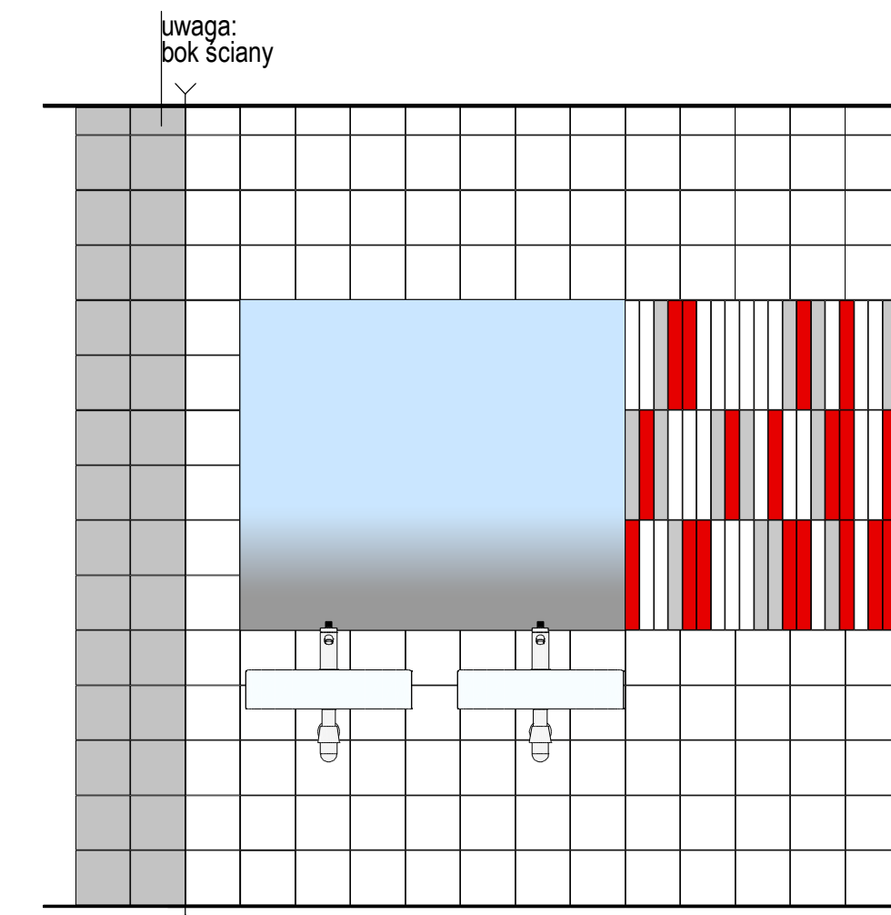
P-04 E-E
