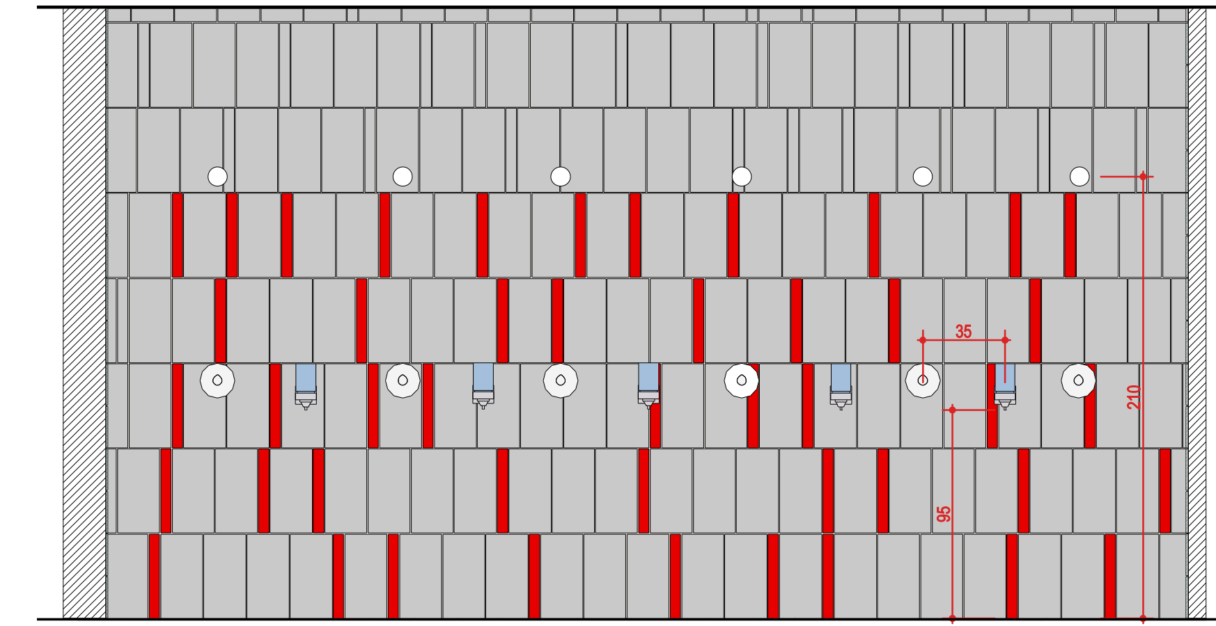
P-04 B-B
