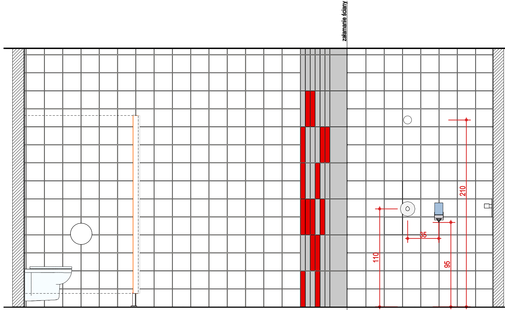
P-04 A-A
