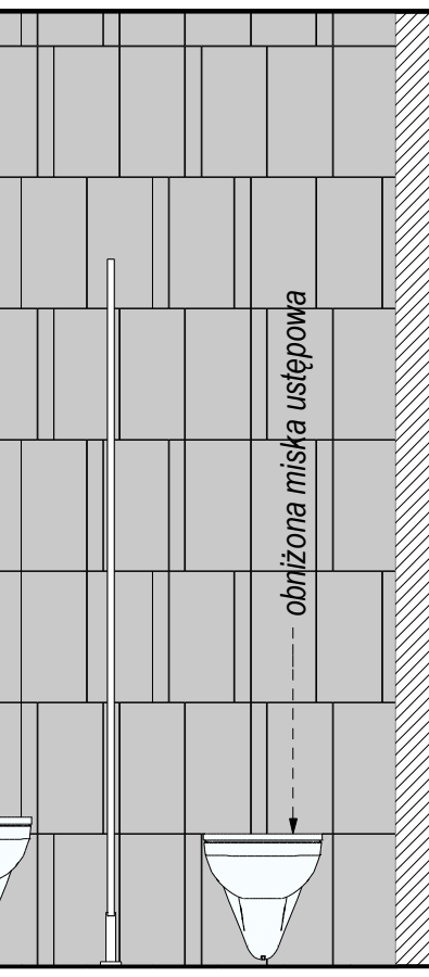
P-04 I-I
