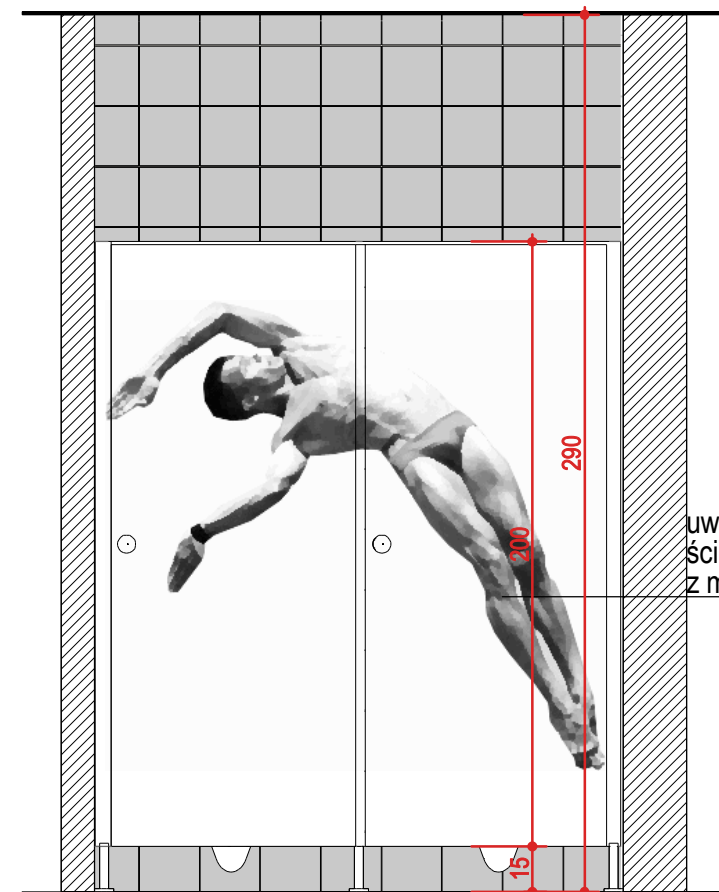
WIDOK ZABUDOWY HPL pomieszczenie 04 natryski K
